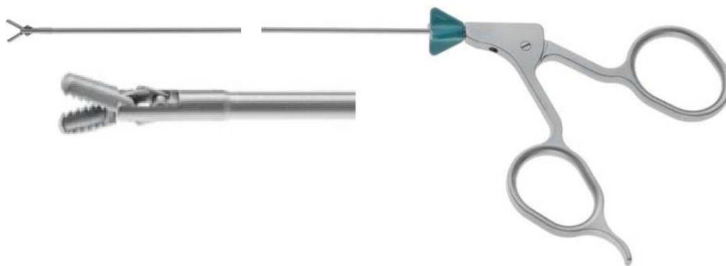
Щипцы эндоскопические захватывающие для крупных камней, с двумя рабочими браншами, длина 600 мм, диаметр 5 Charr., ригидные
